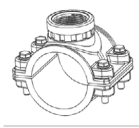
Soporte de sonda para tubo de 63 mm de diámetro, rosca de 1 - 1/4" BL120-575
